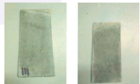
б) пластинки с термодиффузионным цинковым покрытием после удаления коррозии цинкового покрытия
